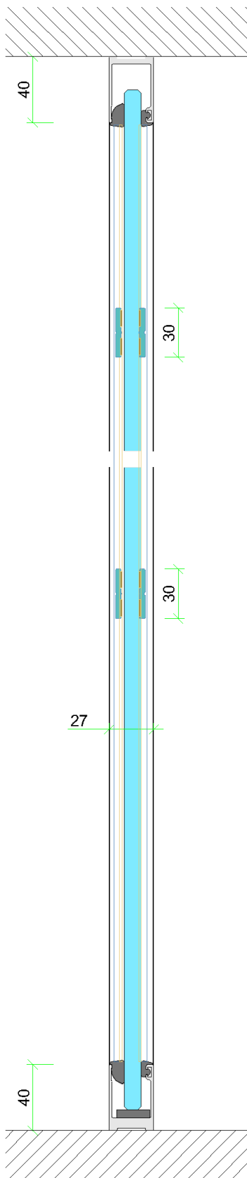
Vertikalschnitt T50 Loft
