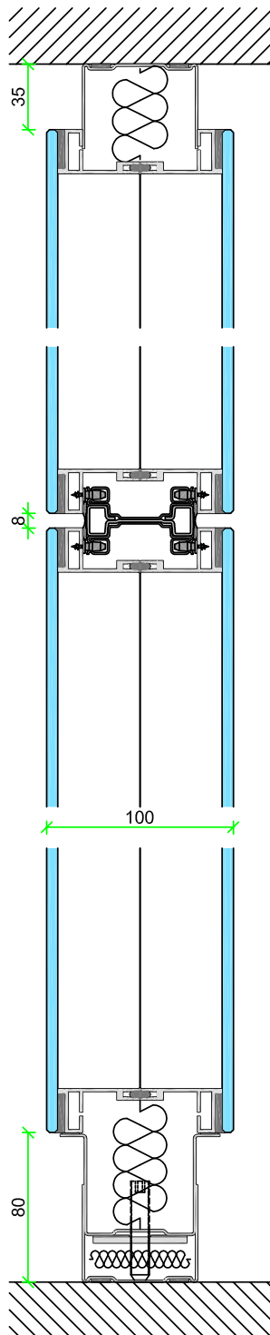
Vertikalschnitt T65
