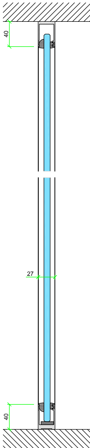
Vertikalschnitt T50
