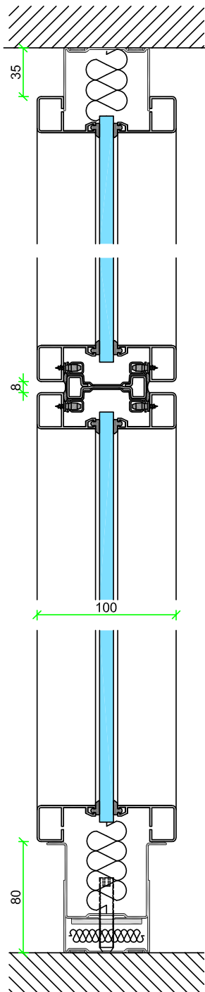
Vertikalschnitt T42
