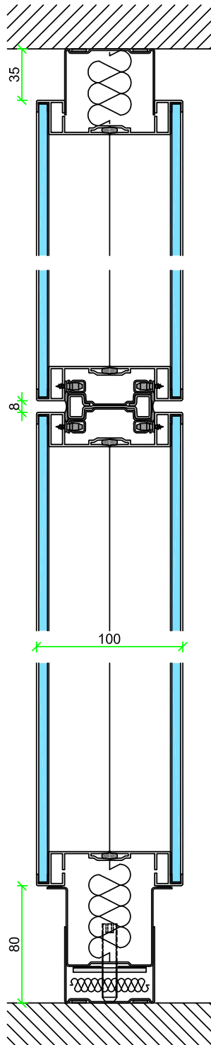
Vertikalschnitt T35
